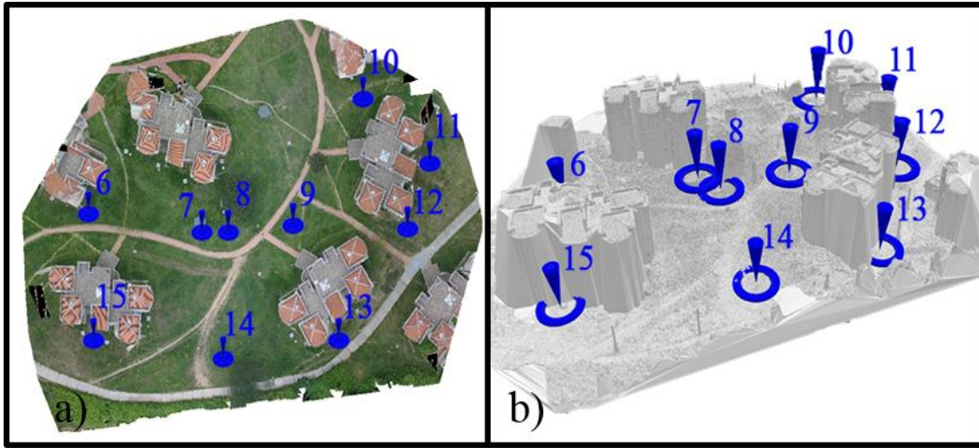
Şekil 4. Gölet öğrenci yurtları YKN'larının a) ortomozaik ve b) sayısal yüzey modeli üzerinde gösterimi.
